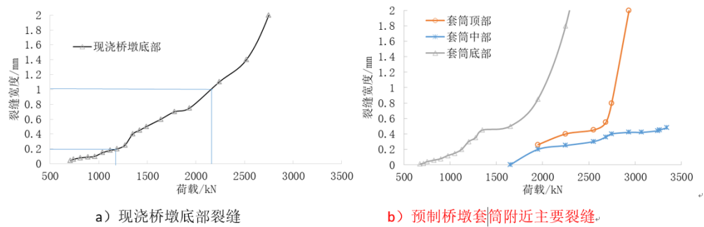
图 8 主要裂缝宽度比较。
