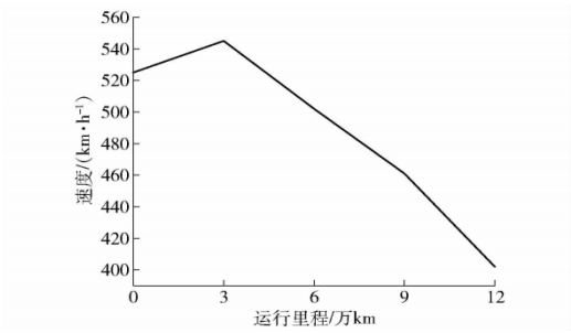
图 8 失稳速度对比 Fig. 8 Comparison of Nonlinear instability velocity
