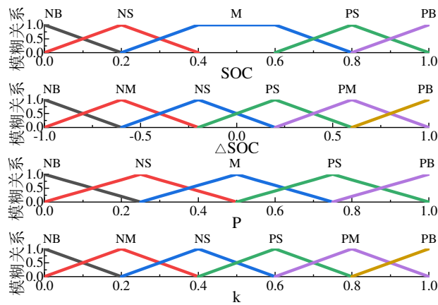
图 A1 模糊控制的隶属度函数
