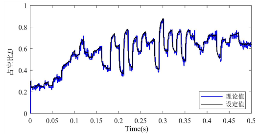
(b) 暂态均值模型结果对比
