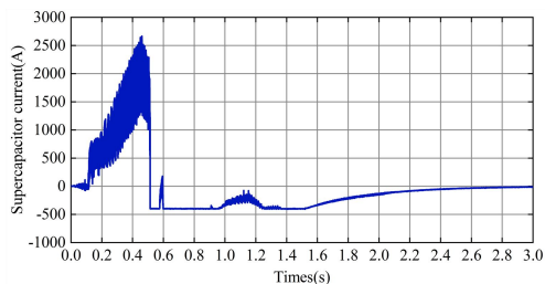
(c) 超级电容输出电流
