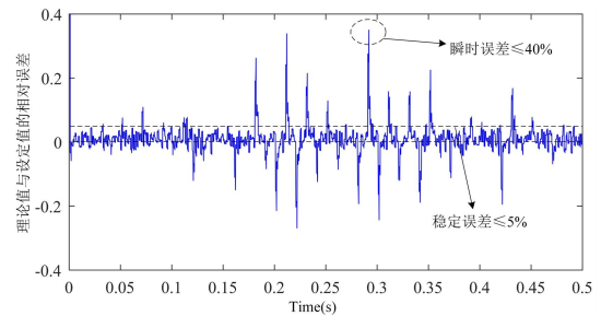
(c) 暂态均值模型误差曲线
