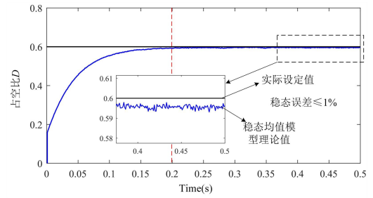
(a) 稳态均值模型结果对比
