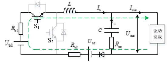
(a) S_1 开通, S_2 关断
