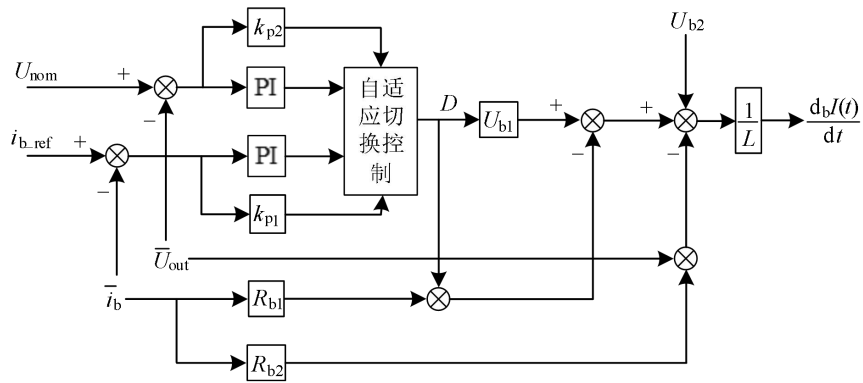
图7 自适应切换控制原理框图
