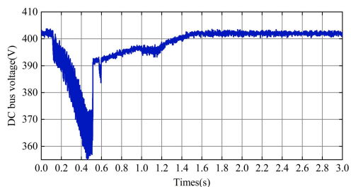
(a) 直流母线电压
