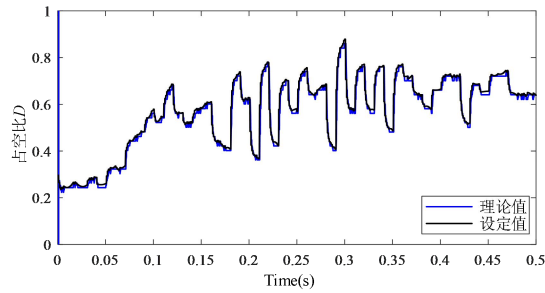
(a) 暂态均值模型结果对比
