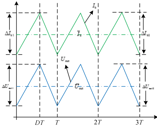
图 3 I_b 与 U_{out} 的稳态波动特性
