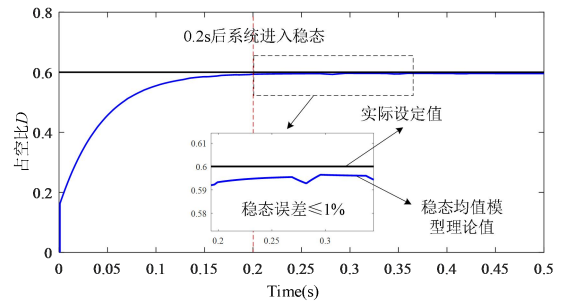
图8 稳态均值模型仿真验证
