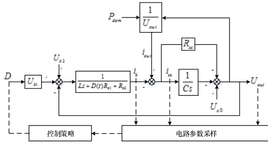
图 6 混合储能系统控制模型
