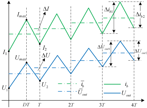
图 5 i_b 与 U_{out} 的暂态波动特性
