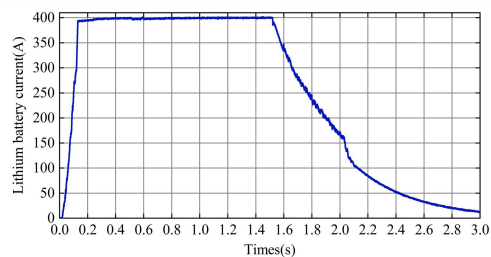
(b) 锂电池输出电流
