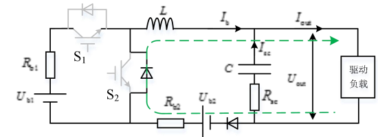
(b) S_1 关断, S_2 开通
