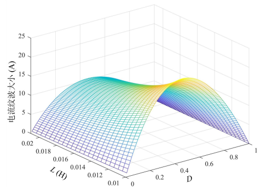
图 4 电流纹波、 D 和 L 的三维关系图
