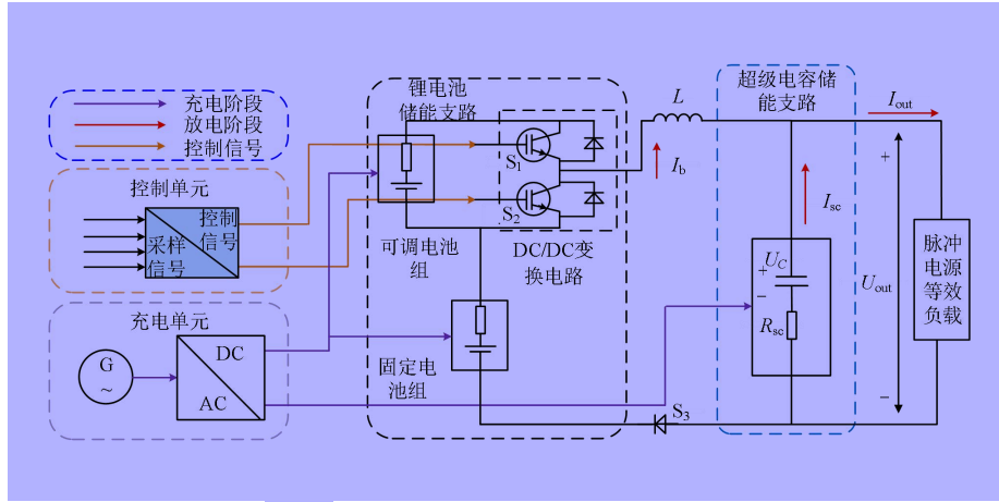
图1 混合储能分组斩波放电拓扑示意图
