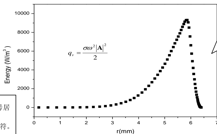
图 2 内热源沿径向的分布
