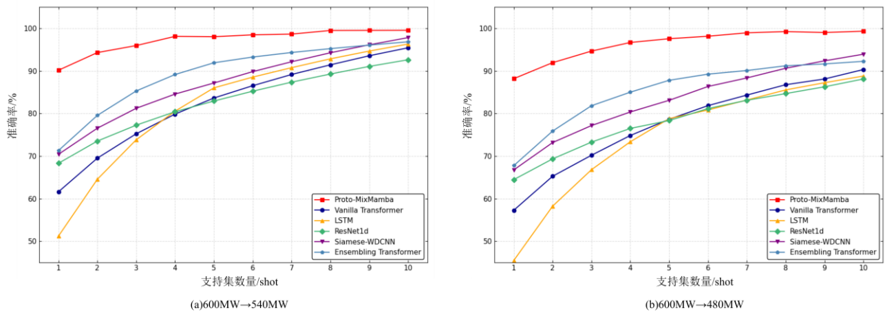
图 4 各模型在不同跨工况少样本任务下的诊断准确率对比
