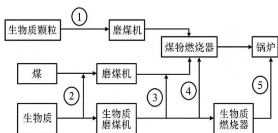
图 8 生物质直接混燃工艺示意图
