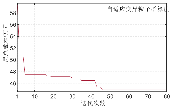
图 4 双层优化模型上层算法收敛曲线
