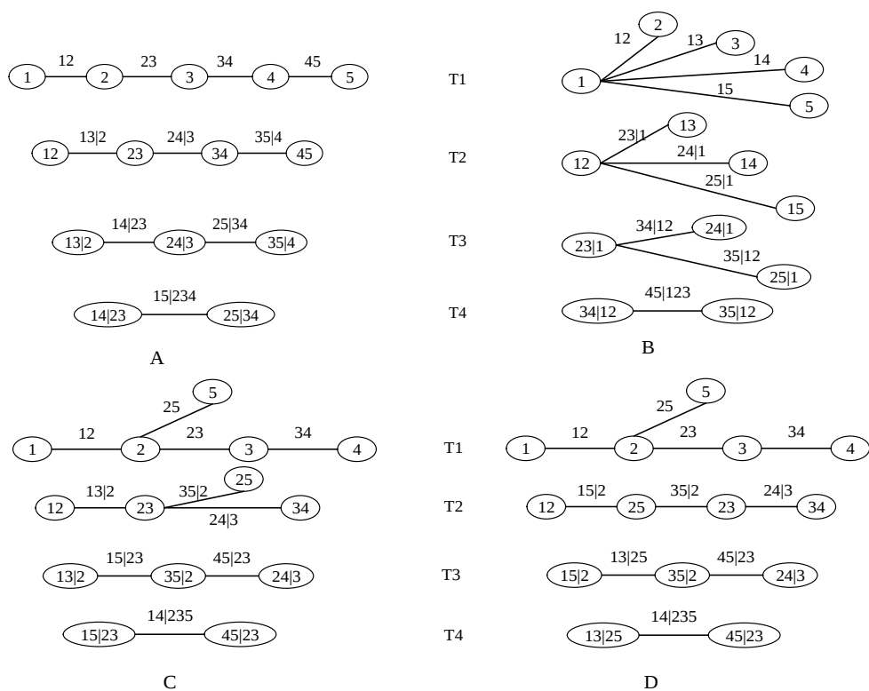
附图 1 5 维 Vine 结构示意图
