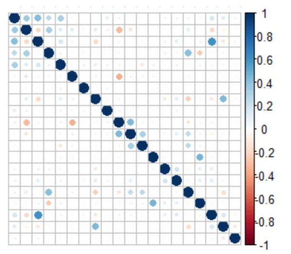
附图 1 解释变量数据的相关性情况（以前 20 个变量为例）
