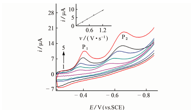
图 1 不同扫速下 M 的循环伏安图 (插图为对应的 i_p - v 线性关系图) (小 5 号黑体)
